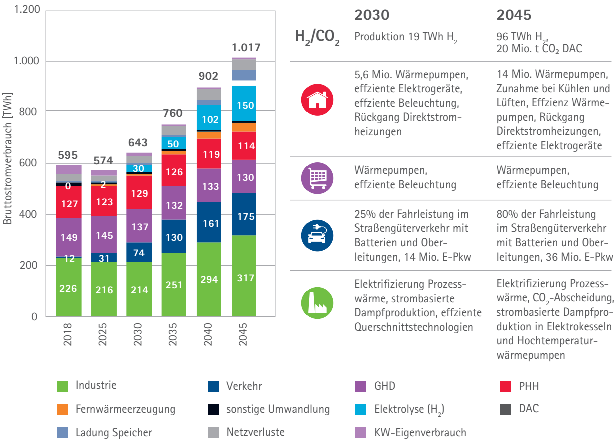
Quelle: Prognos, Öko-Institut, Wuppertal-Institut (2021): Klimaneutrales Deutschland 2045 KW = Kraftwerk. DAC = Direct Air Capture. PHH = Private Haushalte. GHD = Gewerbe, Handel, Dienstleistungen. Verbrauch von Speichern (brutto) beinhaltet Pumpspeicher und stationäre Batteriespeicher in der öffentlichen Versorgung. Der Stromverbrauch von Heimbatterien in Kombination mit PV-Systemen wird hier nicht berücksichtigt.
